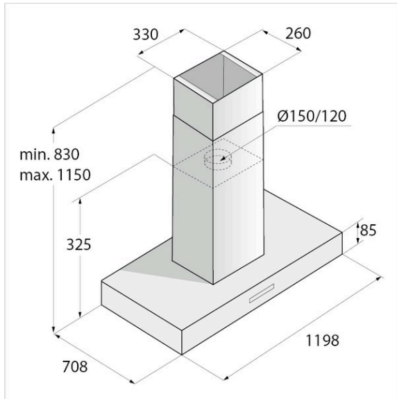
CI41230G Skizze
