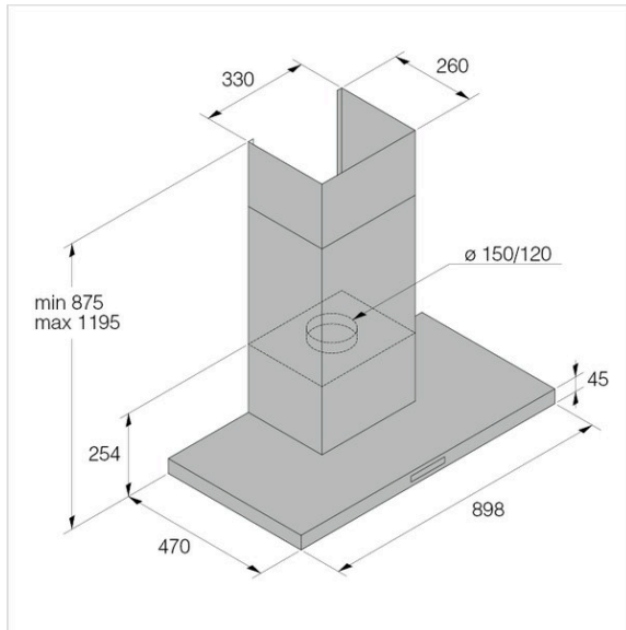
CW4936S Skizze
