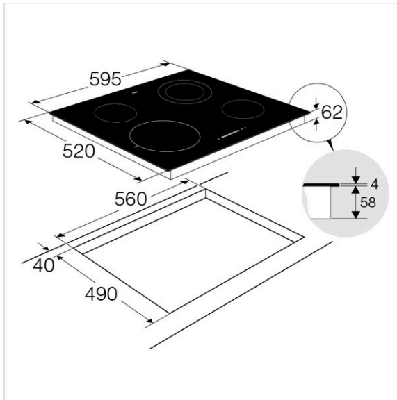
HCL614G Skizze
