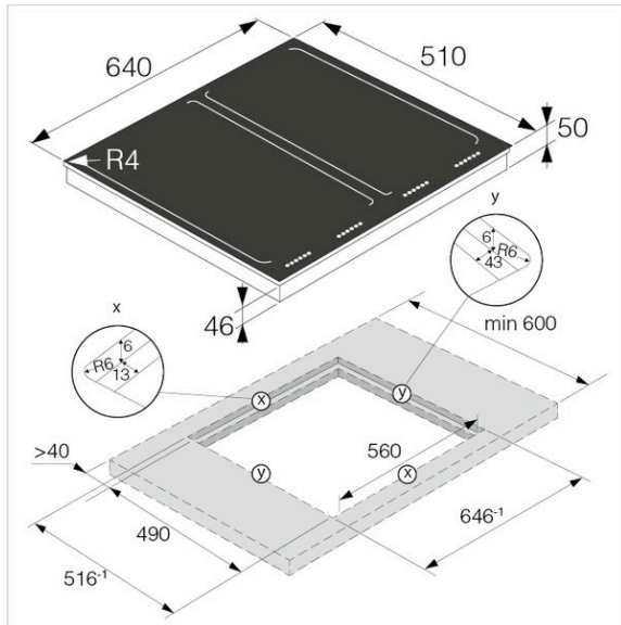
HI1655MF Skizze
