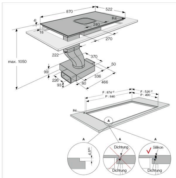
HIHM934M Skizze
