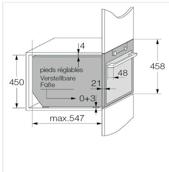
OCM8487A 2 Skizze
