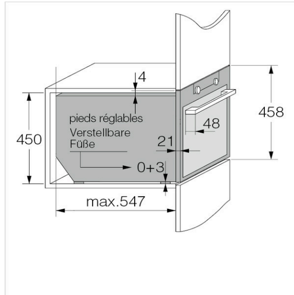
OCM8487A 2 Skizze
