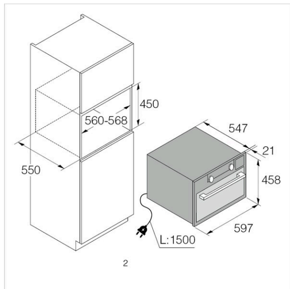
OCS8487S 1 Skizze
