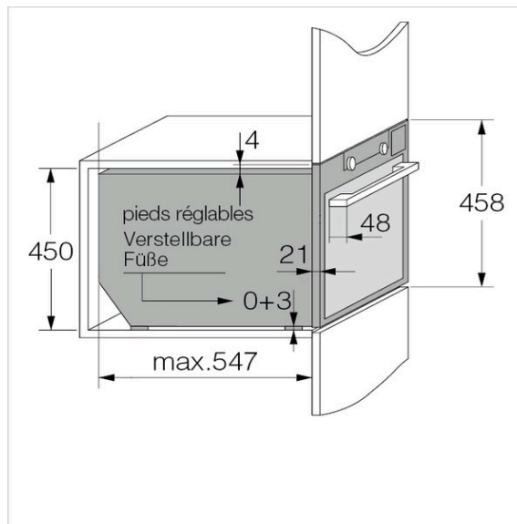
OCS8487S 2 Skizze
