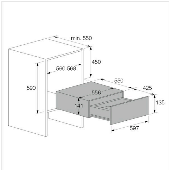
ODV8127S Skizze
