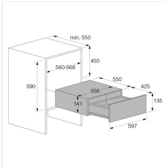
ODV8127A Skizze
