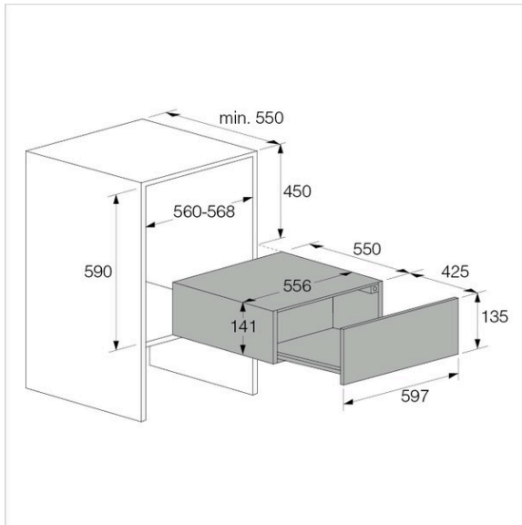
ODW8127S Skizze
