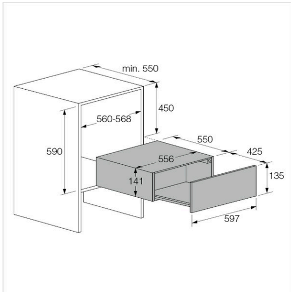
ODW8128G Skizze
